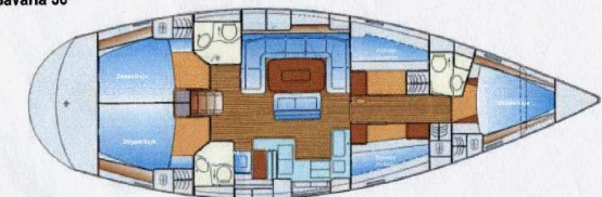
5 Kabinen Grundries
